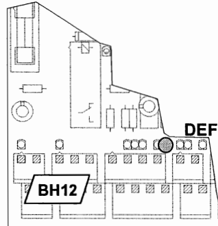
Conséquences d'une erreur de programmation des sorties SPG1, SPG2 et SPG3 (plusieurs fonctions à la même sortie physique)
