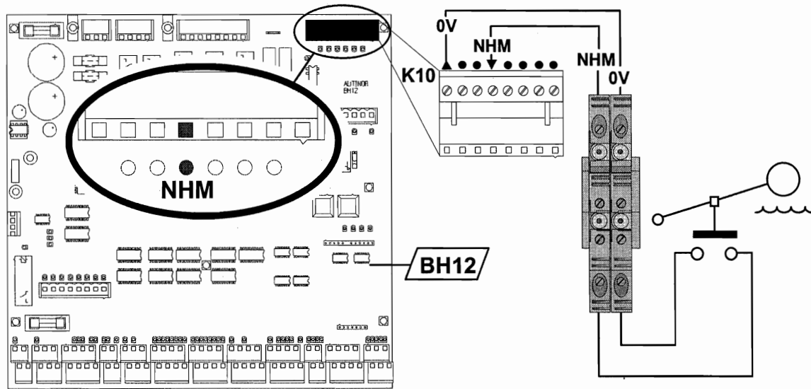
Connexion du contact de « Niveau d'huile minimum »
