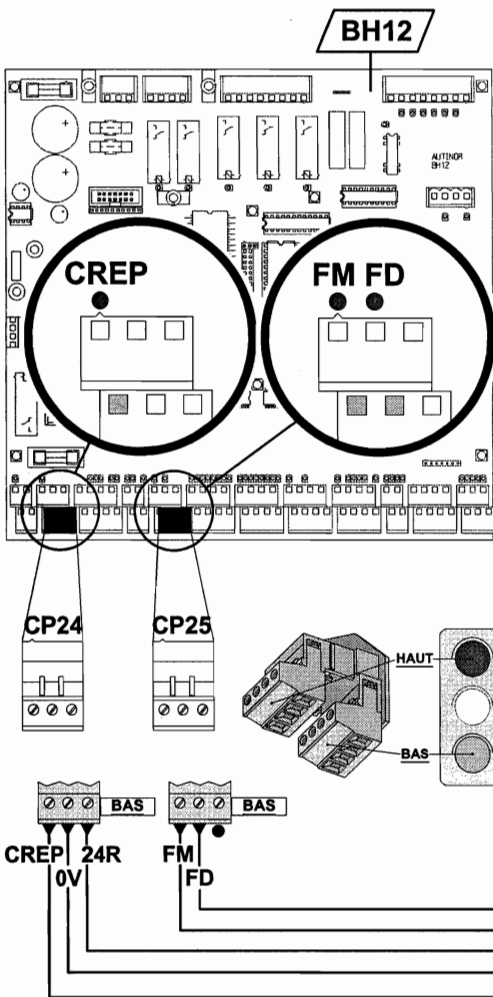
Connexion du répéteur de position au(x) palier(s) modèle IDFL 30/50
