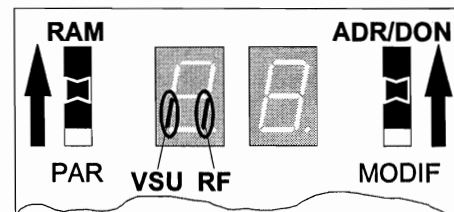
Visualisation du contact, voyant et ronfleur de « Surcharge de la cabine »
