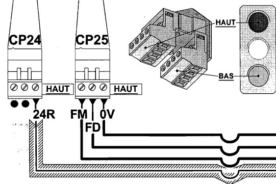
Connexion des flèches de sens en cabine
