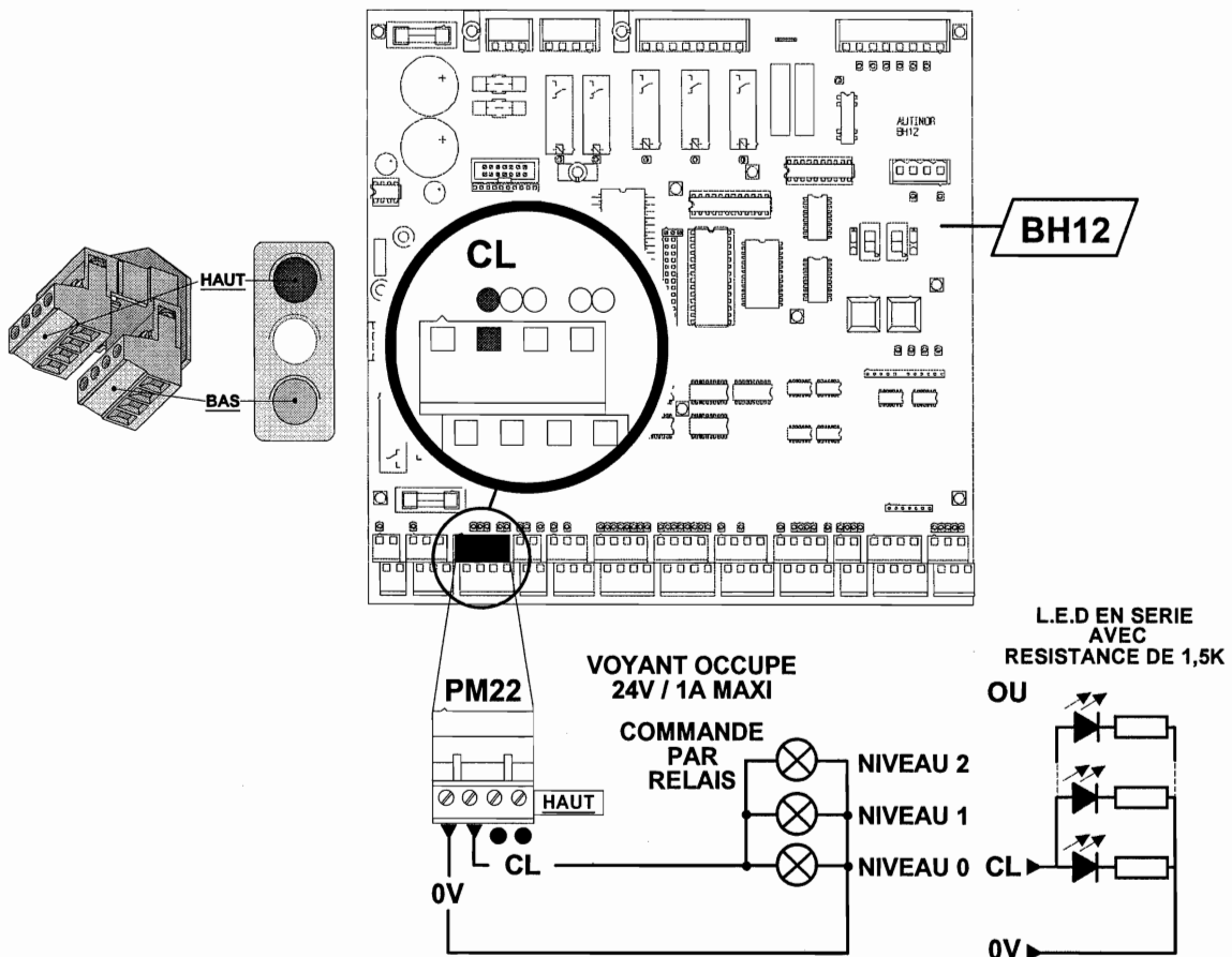
Connexion des voyants « Occupé » aux paliers
