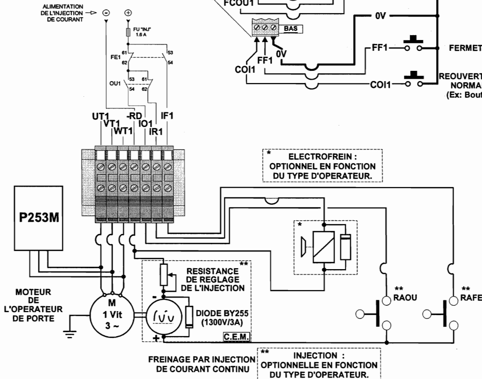
Connexion des contact de l'« Opérateur de porte automatique »
