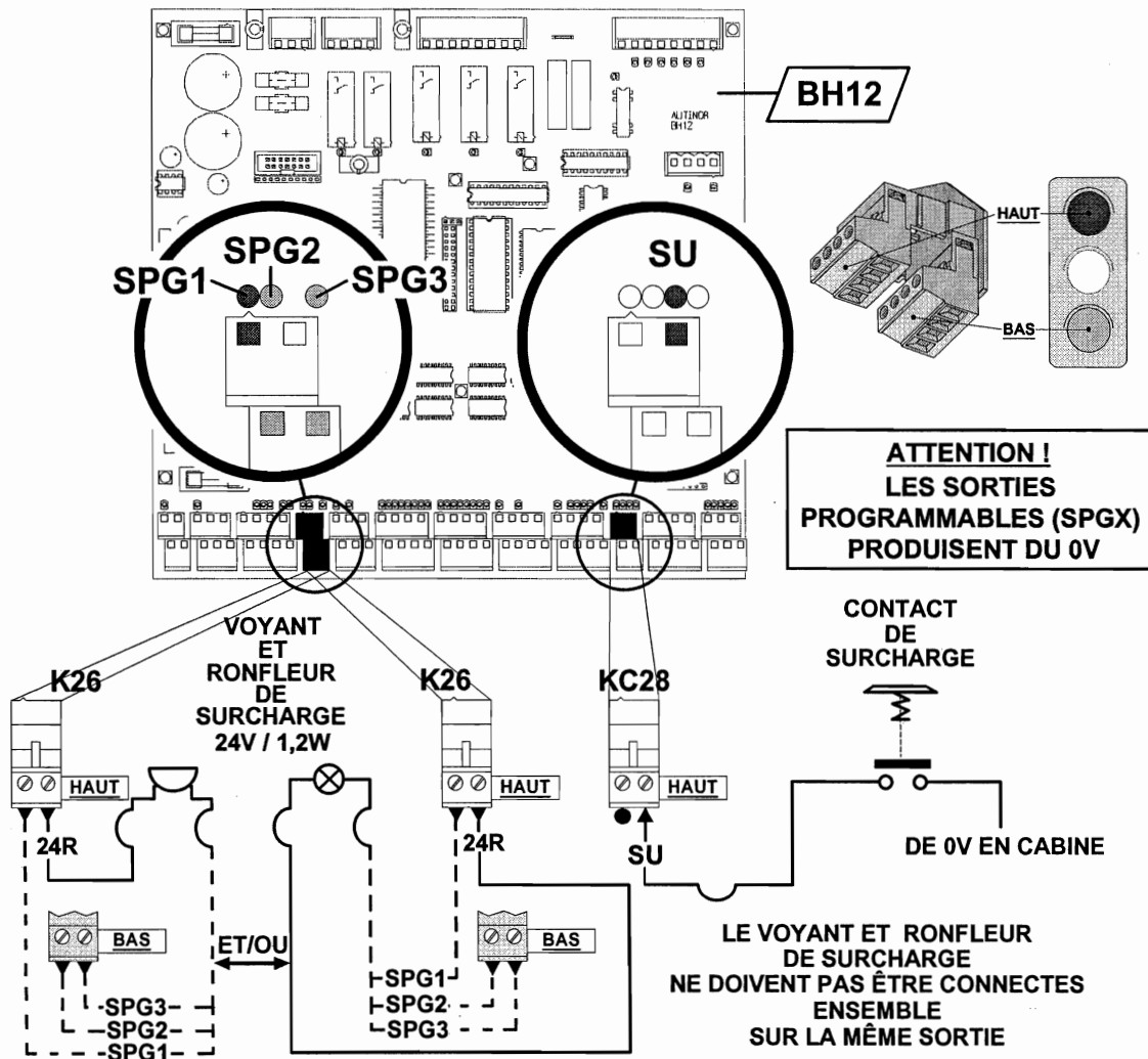
Connexion du contact, voyant et ronfleur de « Surcharge de la cabine »
