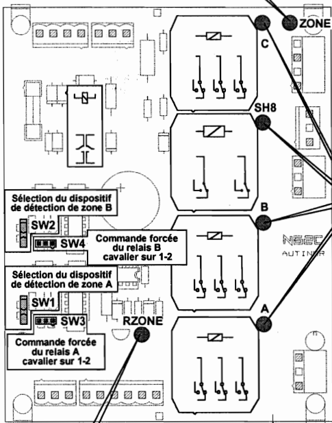
Carte Contrôle de zone de déverrouillage pour antidérive électrique mouv. portes ouvertes
