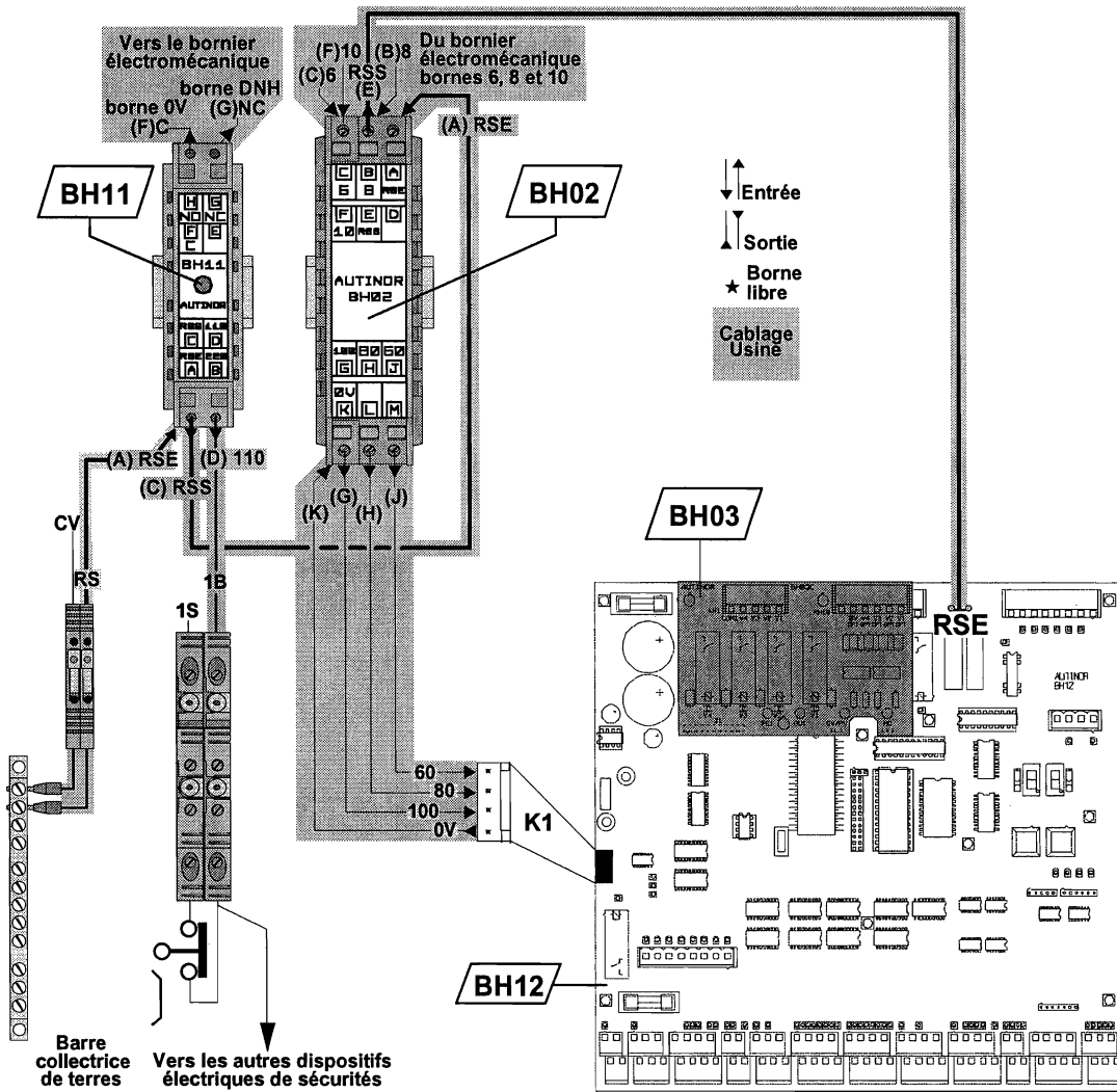
Connexion du contact de fin de course haut
