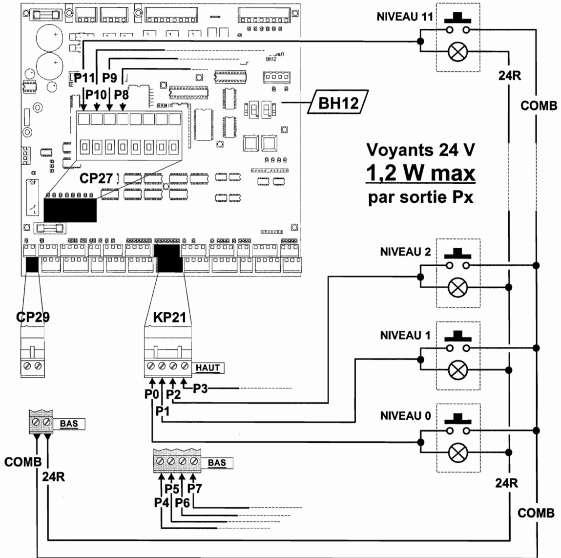
Connexion des boutons d'appel
