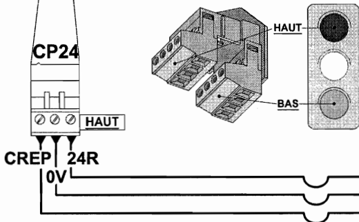
Connexion du répéteur de position en cabine modèle ID 30
