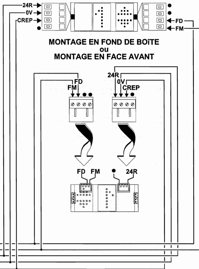
Connexion du répéteur de position au(x) palier(s) modèle IDFL 30/50
