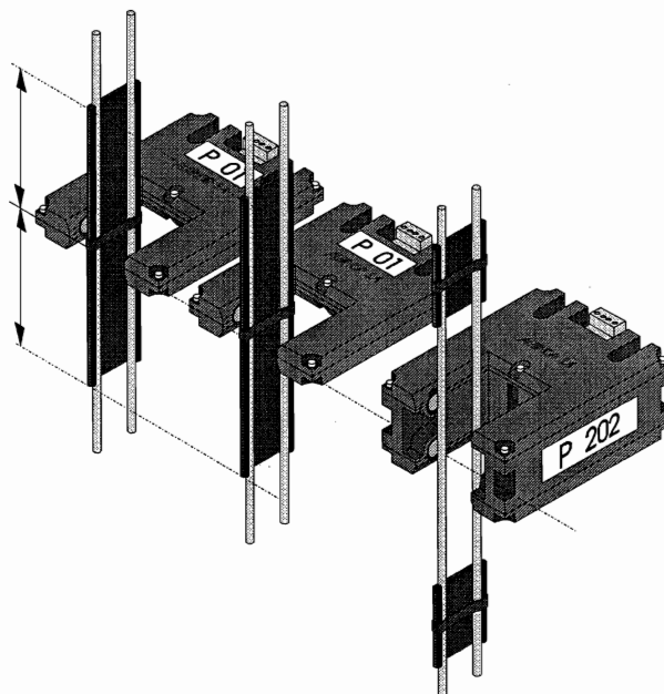
Position des capteurs de zone P01 et de comptage P202
