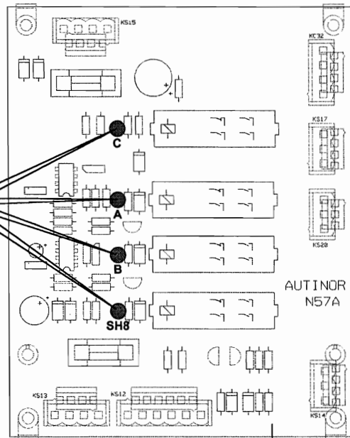
Carte Contrôle de zone de déverrouillage pour antidérive électrique mov. portes ouvertes (Directive Européenne 95/16/CE)
