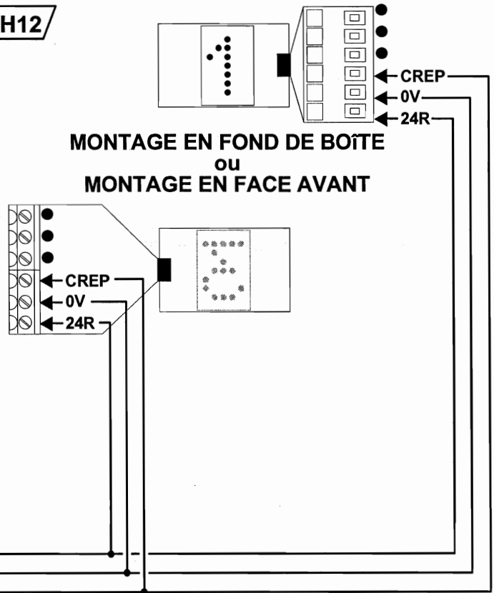
Connexion du répéteur de position au(x) palier(s) modèle ID 50 1 DIGIT
