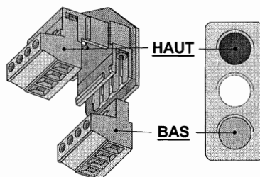
Constitution du connecteur
