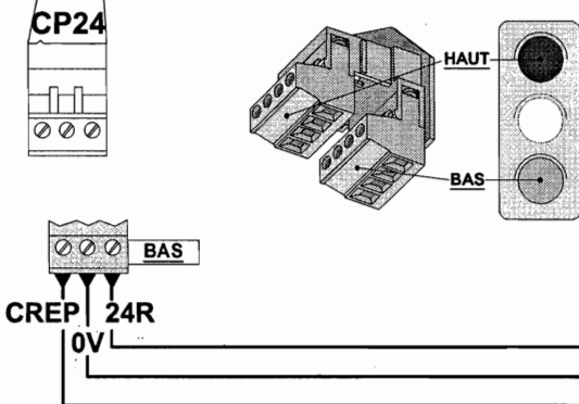
Connexion du répéteur de position au(x) palier(s) modèle ID 50
