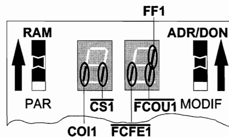
Visualisation de l'état des contact de l'« Opérateur de porte automatique »
