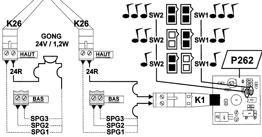
Connexion du gong en cabine
