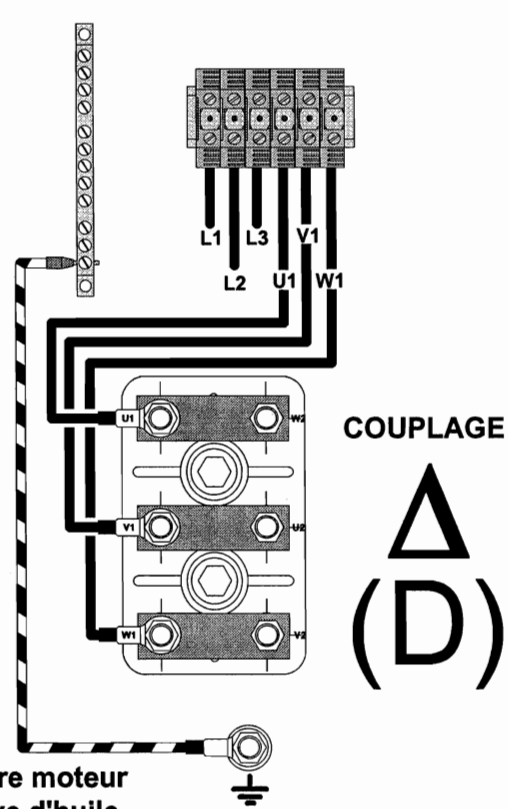
Couplage Triangle Moteur 380 V sur réseau 380 V Moteur 220 V sur réseau 220 V
