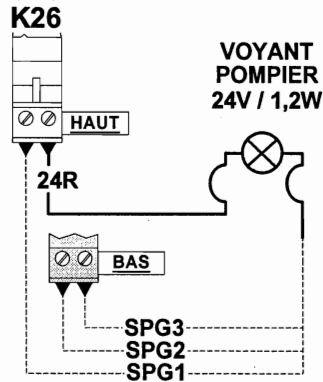
Connexion du voyant pompier
