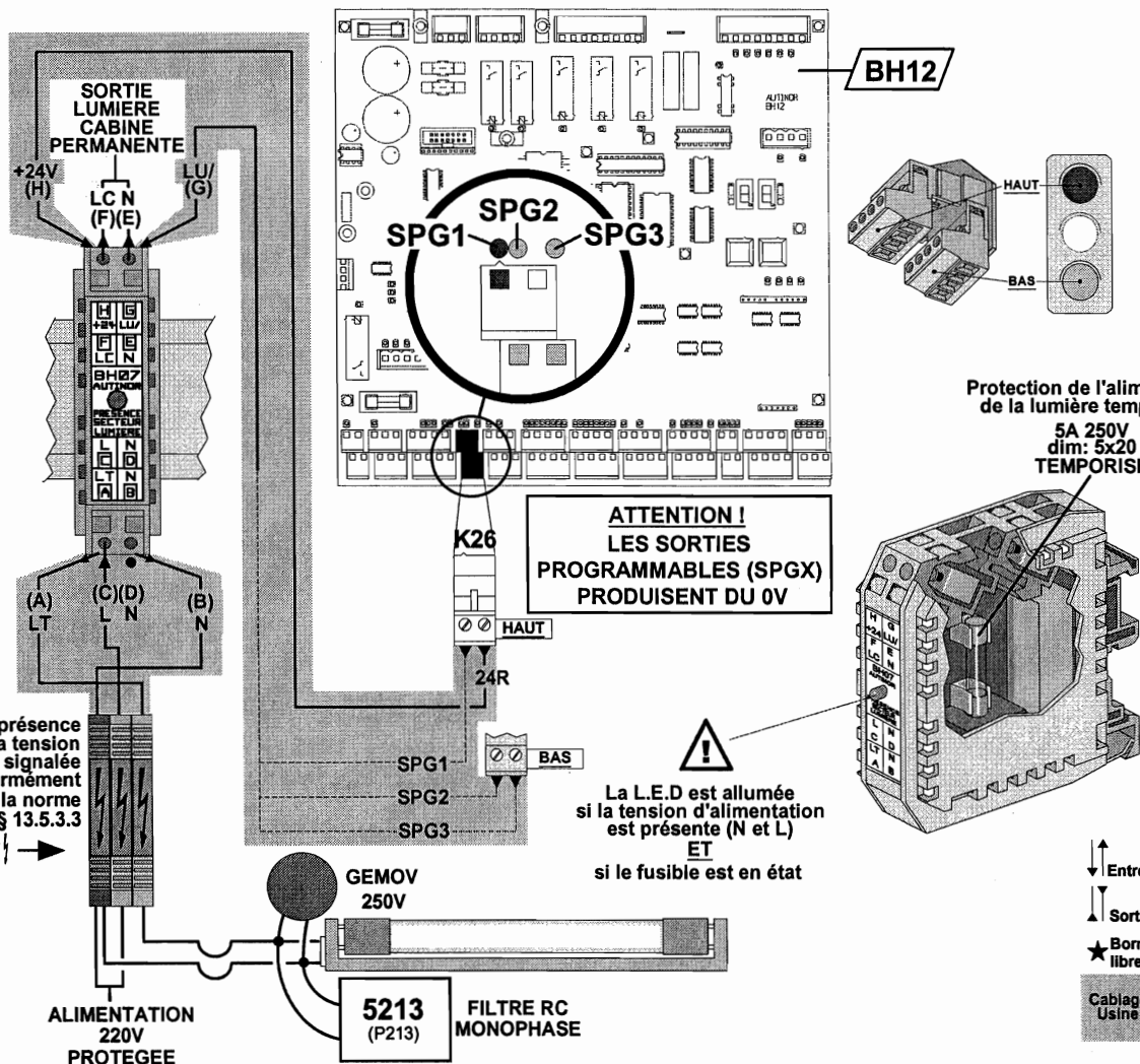
Connexion de la lumière automatique temporisée en cabine
