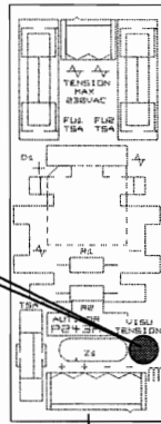
Boîtier et carte Pont redresseur pour transfo TB191
