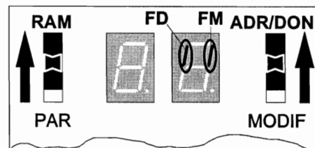
Visualisation de l'état des flèches de sens au(x) palier(s)
