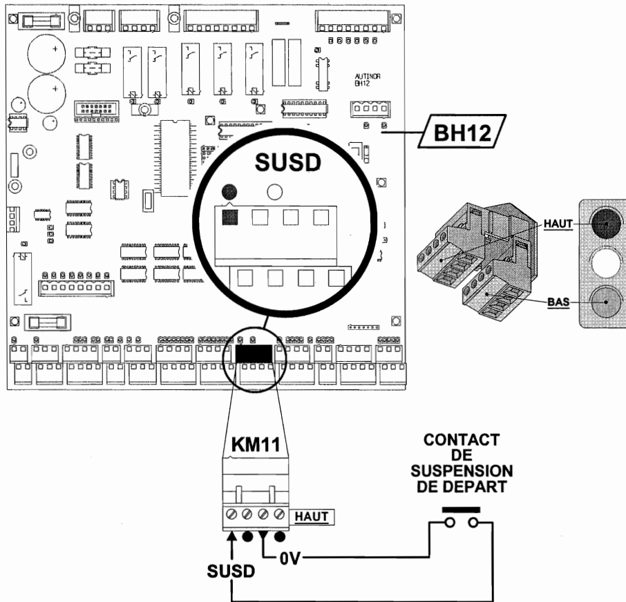
Connexion du contact de « Suspension de départ »
