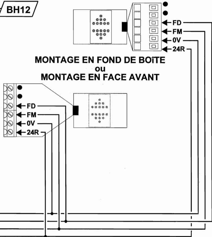
Connexion des flèches de sens au(x) palier(s) modèle FL30 / 50« »
