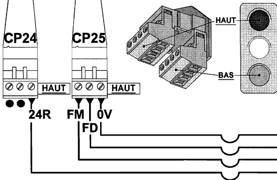
Connexion des flèches de sens en cabine modèle FL30 / 50« »
