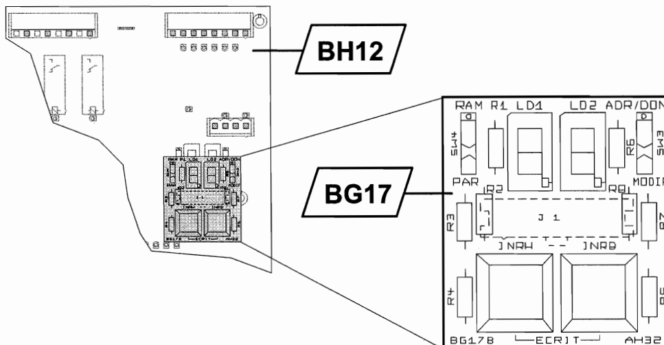
Position des interrupteurs à glissière pour accéder aux paramètres
