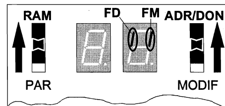
Visualisation de l'état des flèches de sens en cabine modèle FL30 / 50« »
