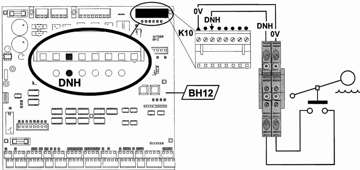
Connexion du contact de « Défaut de niveau d'huile »
