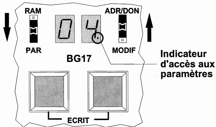
Position des interrupteurs à glissière pour accéder aux paramètres
