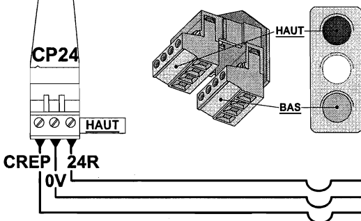
Connexion du répéteur de position en cabine modèle ID 50
