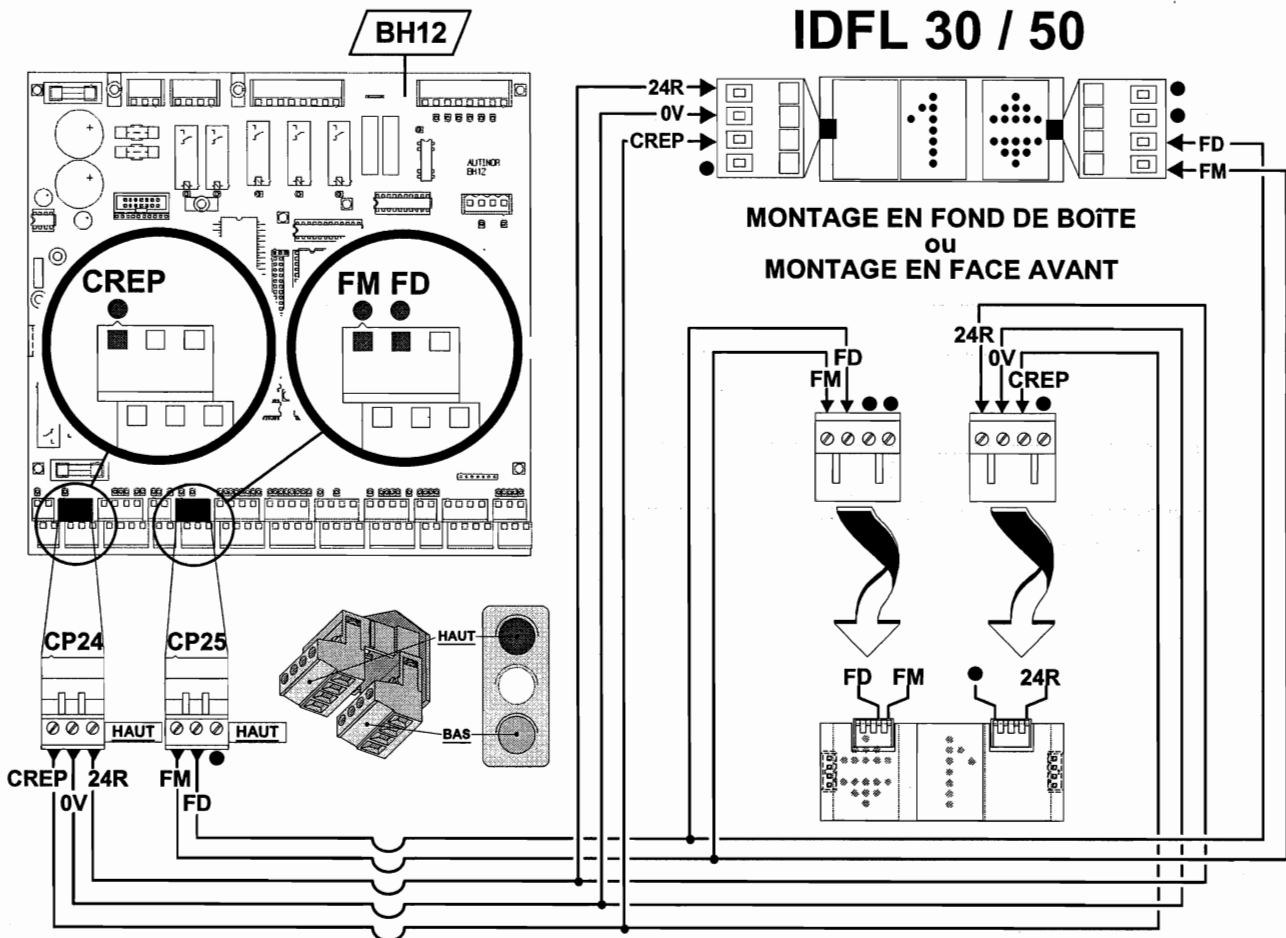
Connexion du répéteur de position en cabine modèle IDFL 30/50
