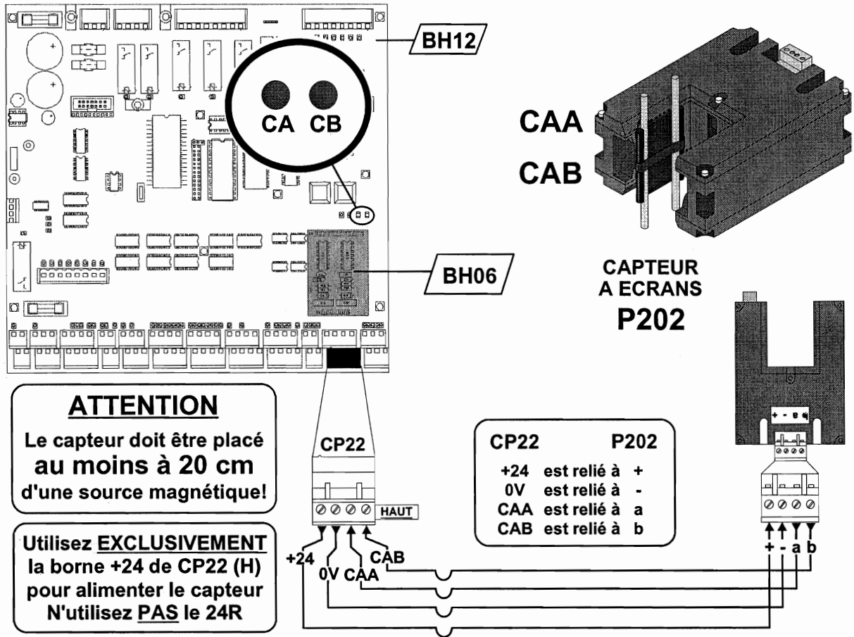
Connexion du capteur P202 (comptage à écrans)
