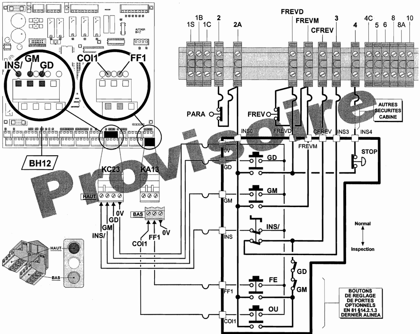
Connexion des contacts de « Manœuvre d'inspection XP P82-511 »
