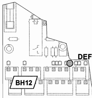
Connexion du voyant pompier
