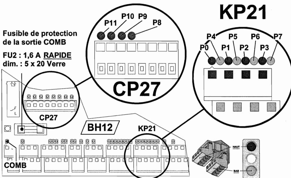
Visualisation de l'état des boutons d'appel
