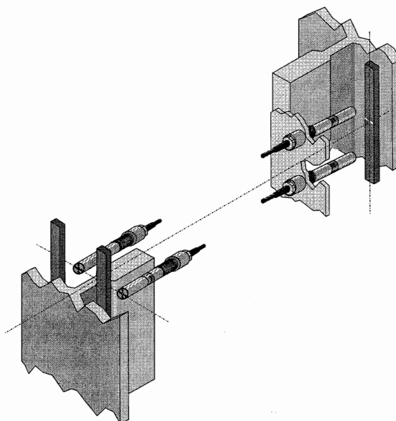
Position des I.L.S. de zone et de comptage
