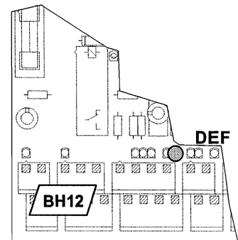
Conséquences d'une erreur de programmation des sorties SPG1, SPG2 et SPG3
