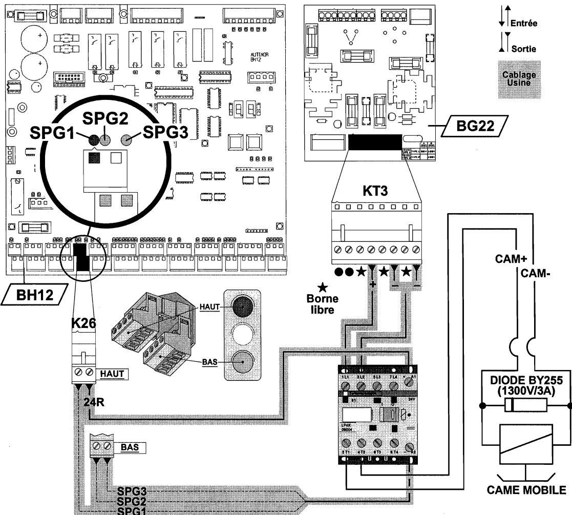
Connexion de la « Came mobile de déverrouillage »
