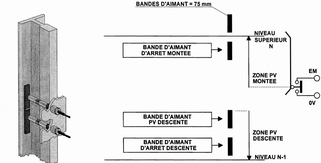
INTERRUPTEURS A LAMES SOUPLES
