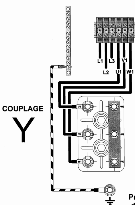
Couplage Étoile Moteur 220 V / 380V sur réseau 380 V
