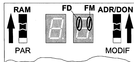
Visualisation de l'état des flèches de sens en cabine
