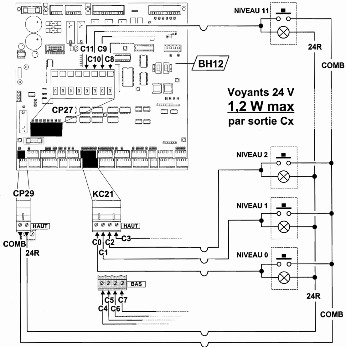
Connexion des boutons d'envoi
