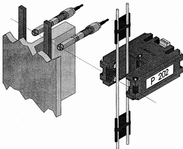
Position des I.L.S. de zone et du capteur de comptage P202
