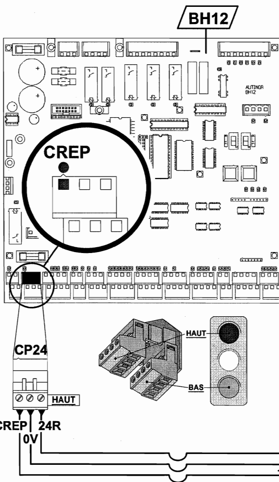
Connexion du répéteur de position en cabine modèle IDFL 30/50 MD
