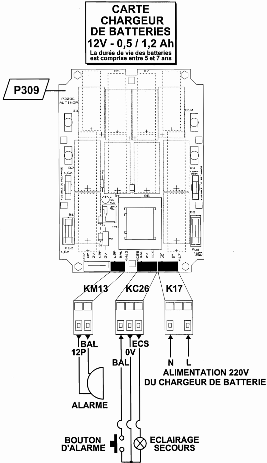
Raccordement du bouton d'alarme
