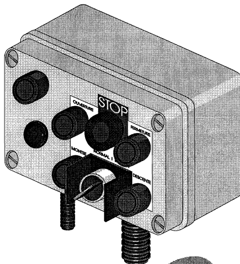
Boîte d'inspection avec boutons de réglage de porte, EN 81 § 14.2.1.3
