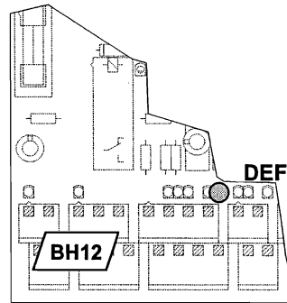
Conséquences d'une erreur de programmation des sorties SPG1, SPG2 et SPG3
