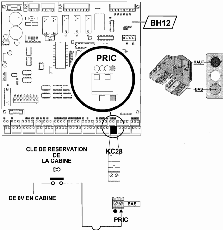
Connexion du contact de « Réservation de la cabine »
