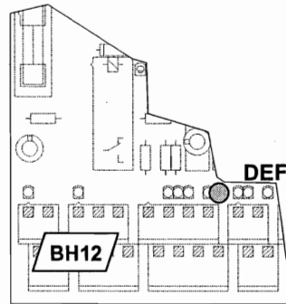
Conséquences d'un collage de durée excessive d'un I.L.S lors du déplacement de la cabine
