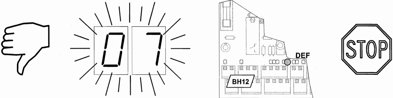
Conséquences d'une erreur de programmation des sorties SPG1, SPG2 et SPG3 (plusieurs fonctions à la même sortie physique)
