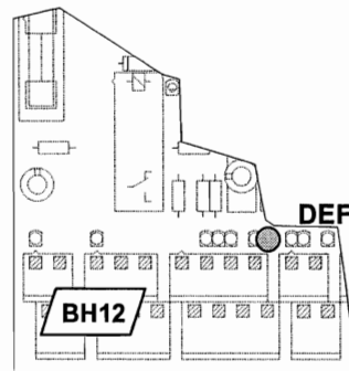
Conséquences d'une coupure simultanée des contacts Extrême Montée et Descente
