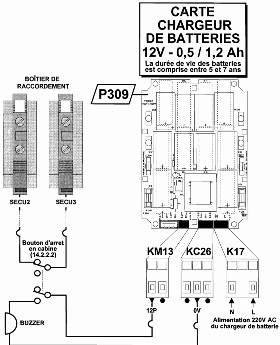
Raccordement du bouton d'arrêt en cabine
