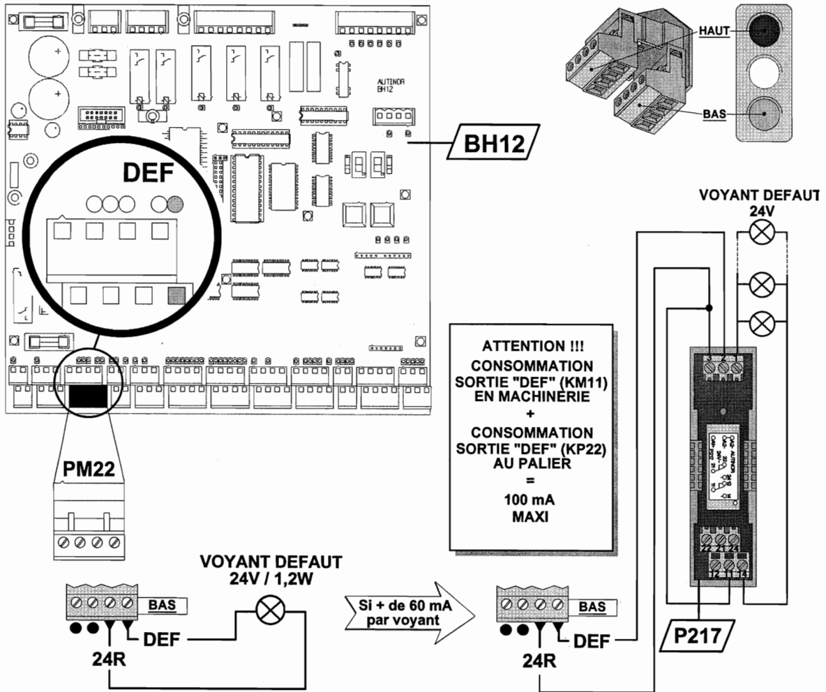
Connexion du voyant défaut
