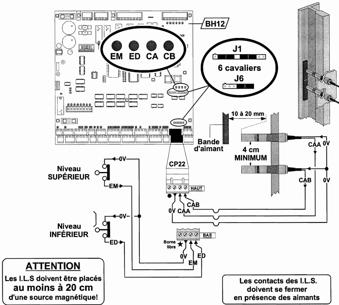
Connexion des I.L.S. et des contacts extrêmes
