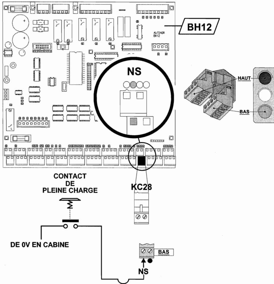
Connexion du contact de « Pleine charge »
